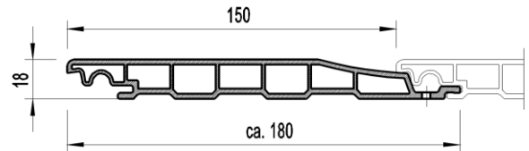
vinylPlus Stülpprofil
