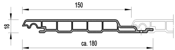
vinylPlus Rundprofil
