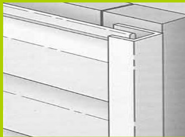
U-Einfassprofil für seitlichen, oberen u. unteren Abschluß
