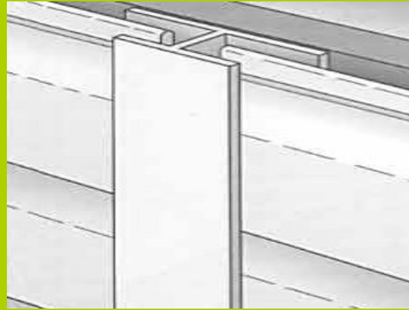
Stossverbindungsprofil bei Längen über 6,00 m
