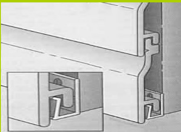
Montagebeispiel für waagerechte Verlegung
