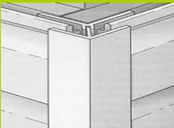
Außeneckprofil mit verdeckter Schnittkante
